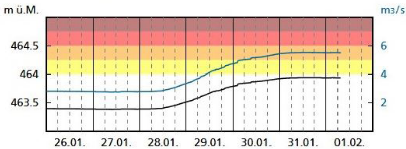
Grafik Abfluss und Wasserstand des Aabachs, Messstation Richensee
