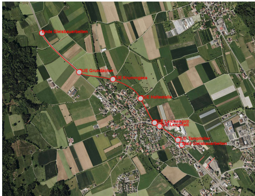
Abbildung: Abschnitt Gleisbauarbeiten mit 6 Bahnübergängen (Quelle: Geportal Kanton Luzern)
